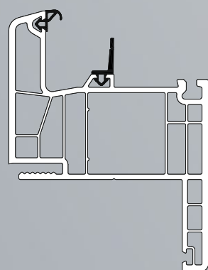
Profil ramă renovare S.80111
