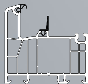
Profil ramă S.80101
