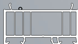
Profil adăugare ramă S.80702
