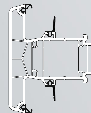
Profil montant S.80301
