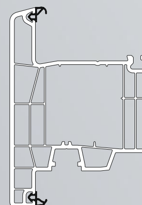
Profil cercevea ușă deschidere exterioară S.80212
