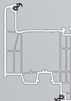
Profil cercevea ușă deschidere interioară S.80211
