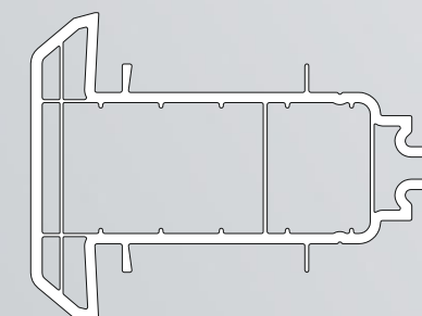
Profil cuplare statică 606-06
