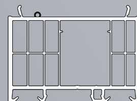
Profil adăugare ramă S.80703
