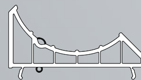
Profil adaptor țevă S.80604
