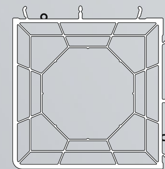
Profil cuplare 90° S.80605
