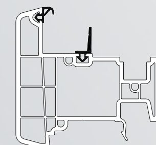
Profil montant mobil S.80401
