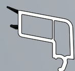
Profil baghetă S.80501
